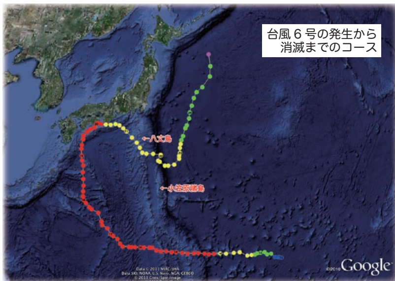
台風発生からの八丈島における気象データ
